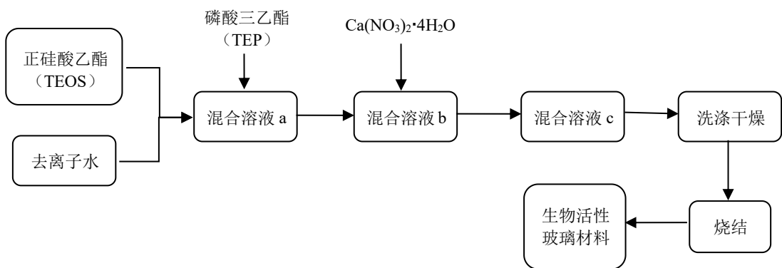
图 2-4 生物活性玻璃生产工艺流程图
