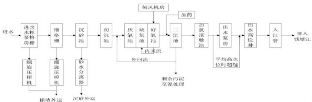
图 4-1 杭州七格污水处理厂废水处理工艺流程图
