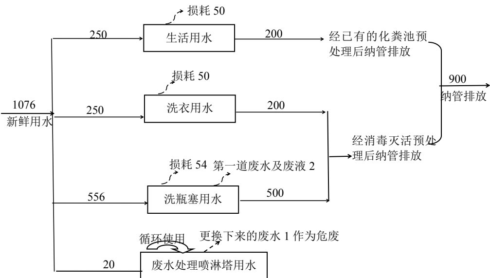
图 2-2 项目用水平衡图 单位：t/a
