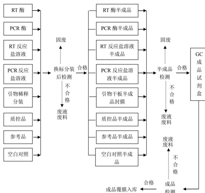
图 2-1 项目核酸试剂盒生产工艺流程图
